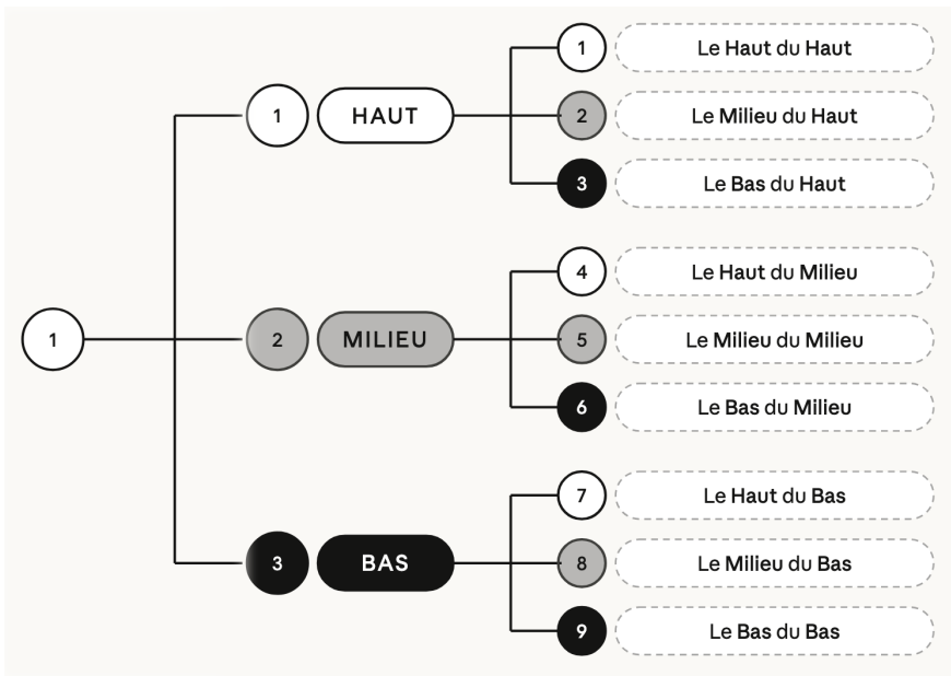
Figure 2 : l'Arbre Ternaire
